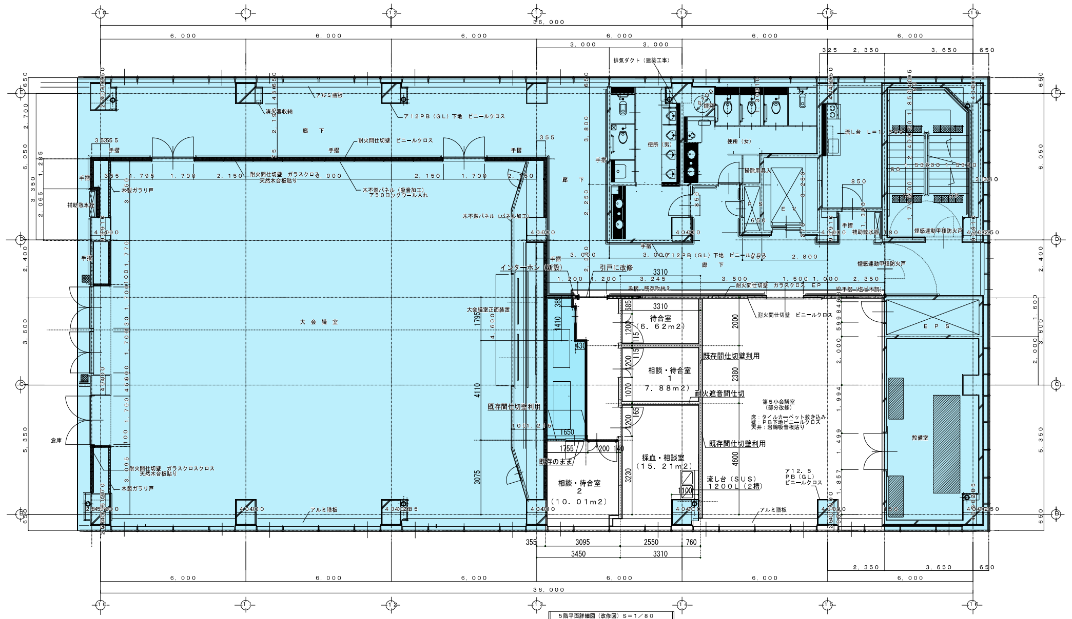
5階平面詳細図 (改修前) S=1/80
