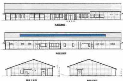
清水支所立平面図
