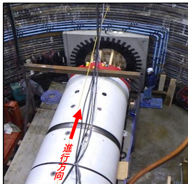
シールド掘削機：内径φ1800mm (先端部)
