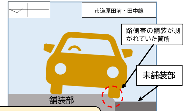
事故発生状況(断面図)
