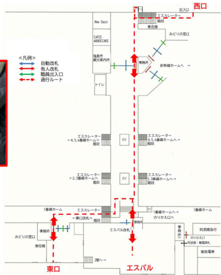
平面図
