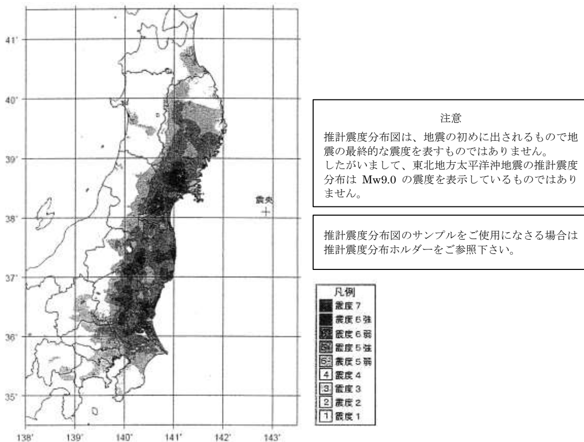
東北地方太平洋沖地震の推計震度分布図（出典：気象庁）
