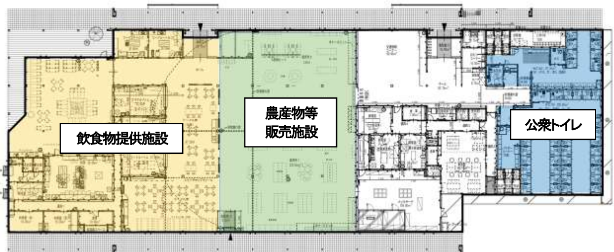
(6) 道の駅本体 平面図
