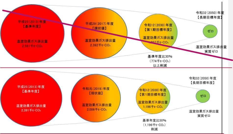
図4-2-1 本市の温室効果ガス排出量削減目標
