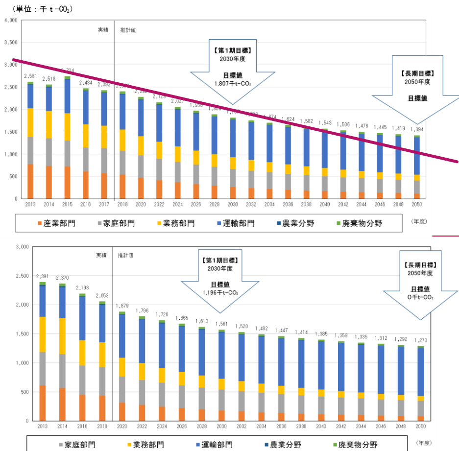
図 4-3-1 温室効果ガス排出量将来推計値
