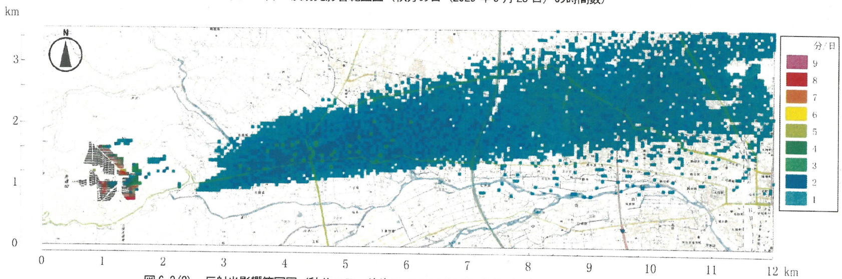
図 6-3(2) 反射光影響範囲図（秋分の日前後 10 日間（2025 年 9 月 13～10 月 3 日）の最大日の時間数）
