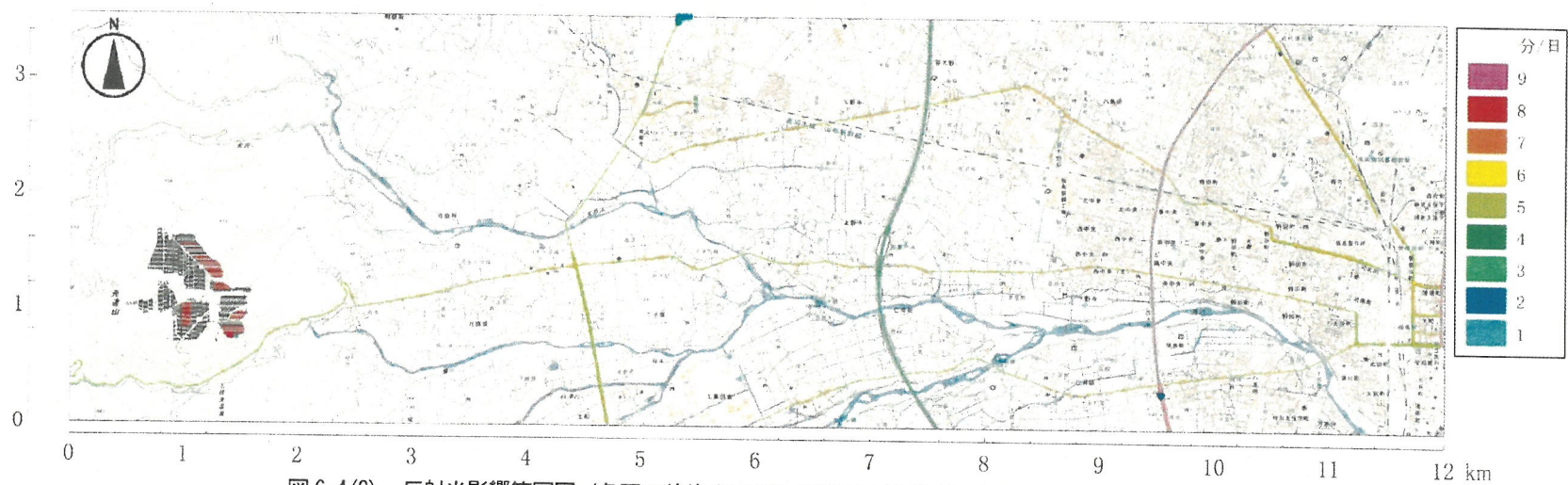
図 6-4(2) 反射光影響範囲図 (冬至の前後 10 日間 (2025 年 12 月 12~1 月 1 日) の最大日の時間数)
