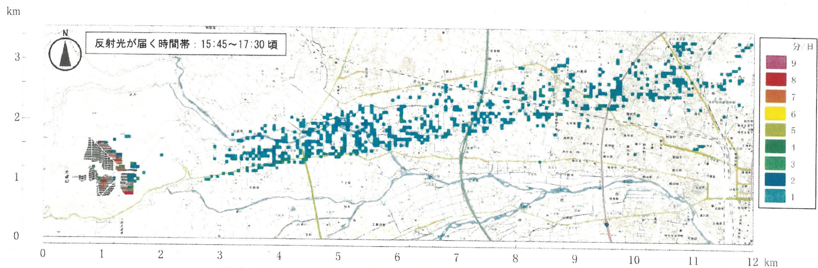
図 6-3(1) 反射光影響範囲図（秋分の日（2025 年 9 月 23 日）の時間数）
