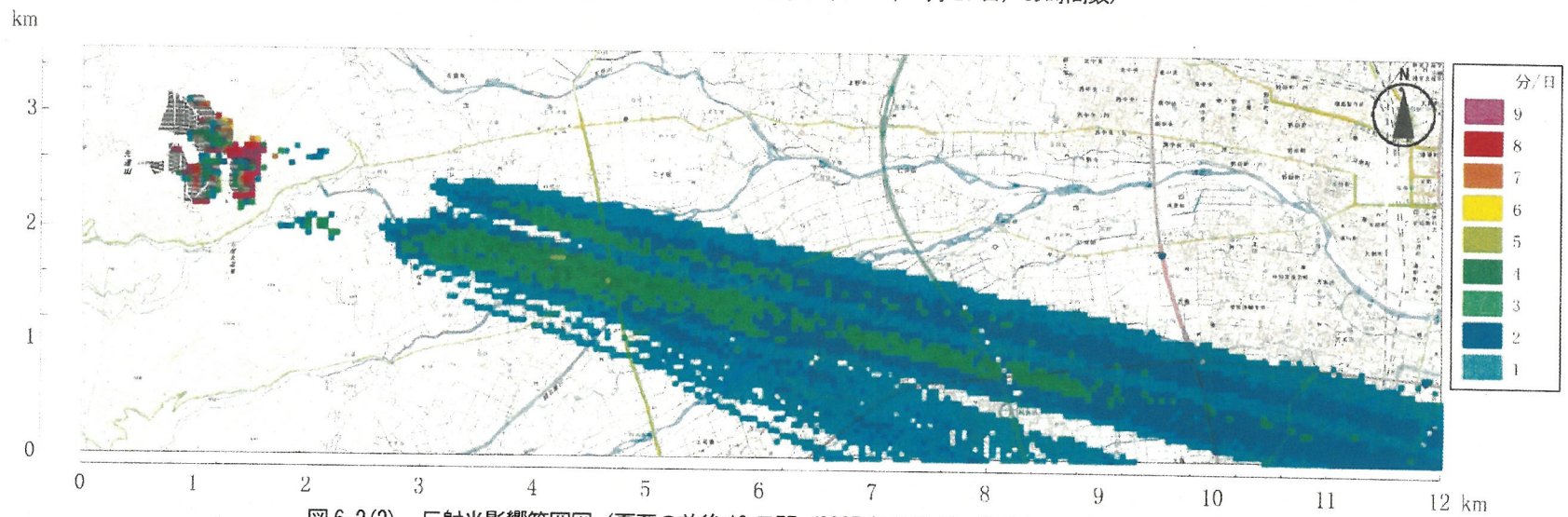
図 6-2(2) 反射光影響範囲図（夏至の前後 10 日間（2025 年 6 月 11～7 月 1 日）の最大日の時間数）
