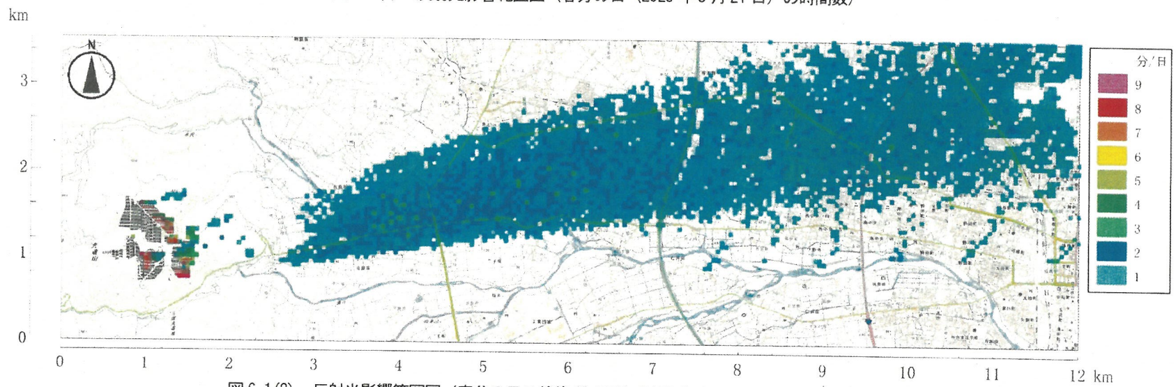
図 6-1(2) 反射光影響範囲図（春分の日的前後 10 日間（2025 年 3 月 10～30 日）の最大日の時間数）
