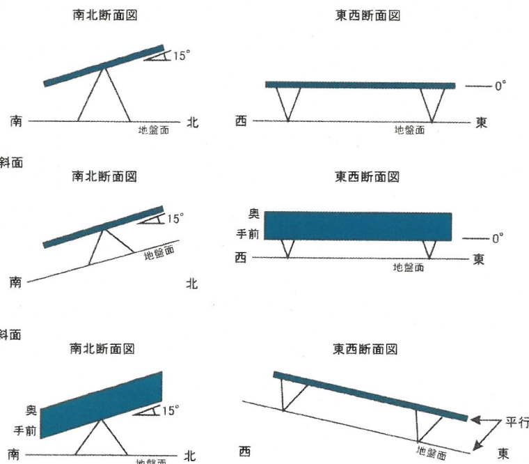
図2 アレイ群の向きの説明図
