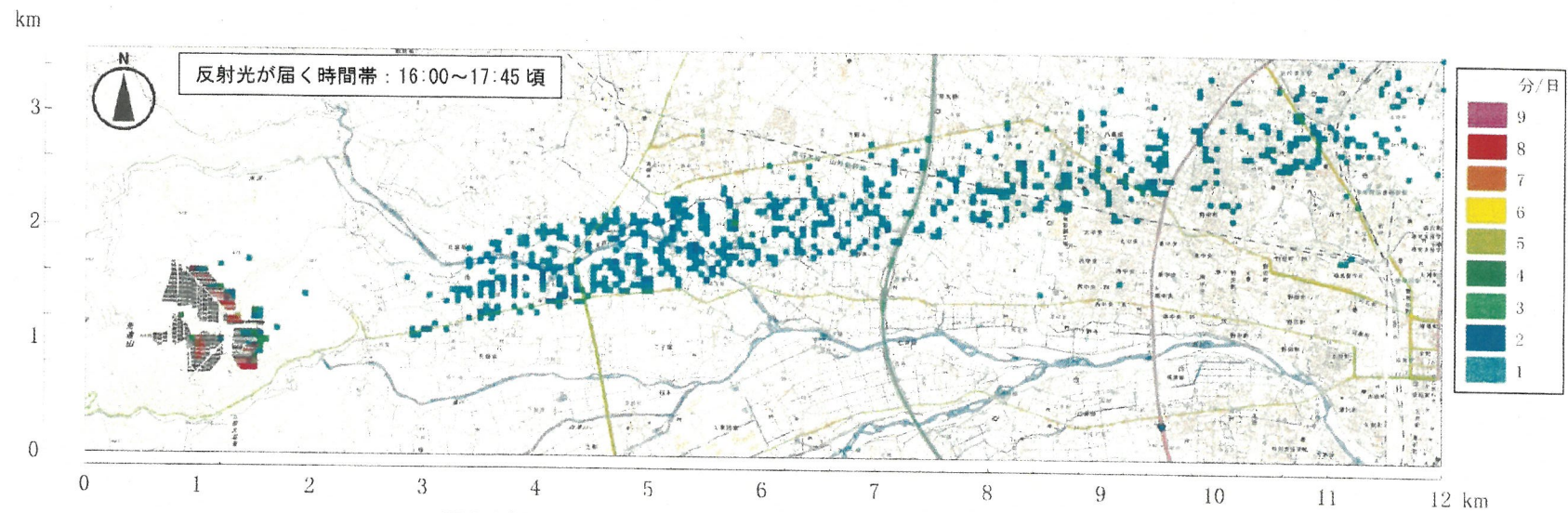
図 6-1(1) 反射光影響範囲図（春分の日（2025 年 3 月 21 日）の時間数）
