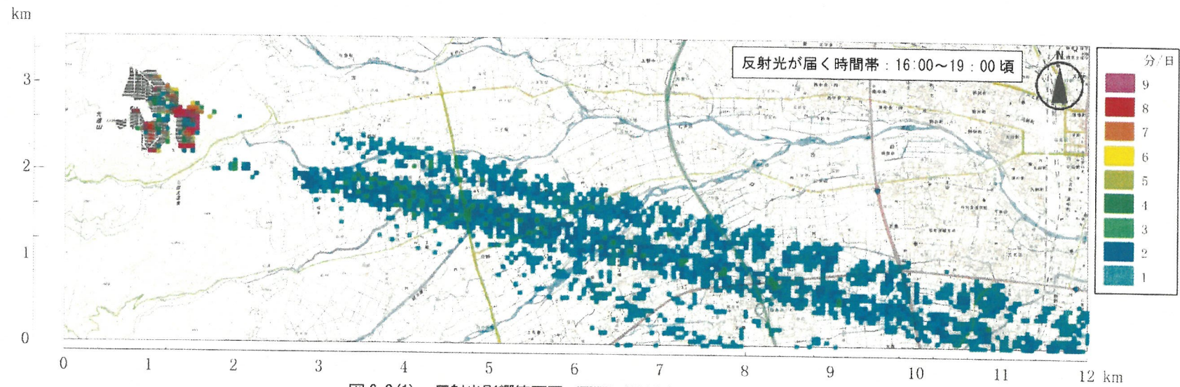
図 6-2(1) 反射光影響範囲図（夏至（2025 年 6 月 21 日）の時間数）
