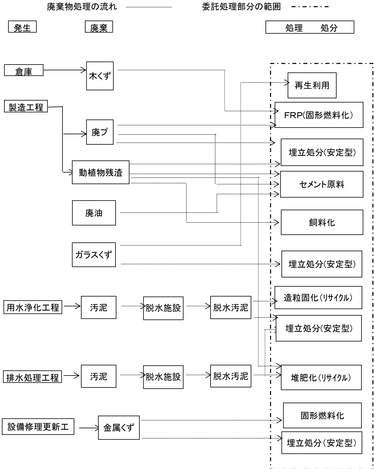
別紙1: 廃棄物処理フロー図(現状)
