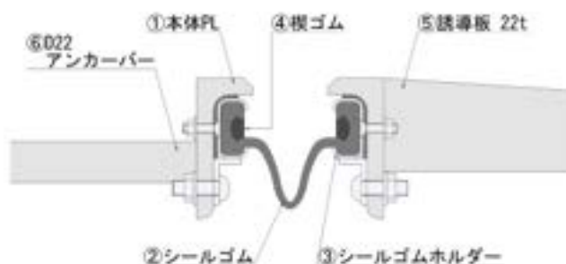
伸縮装置（HK-200007-A）
