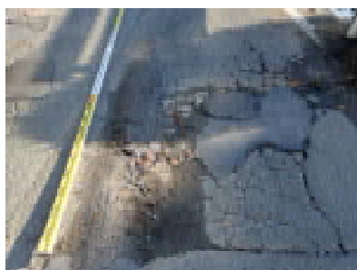
舗装のひびわれ・ポットホール
