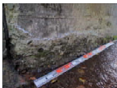
橋台の洗堀
