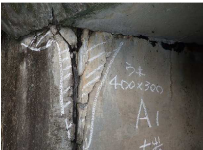
橋台のうき
