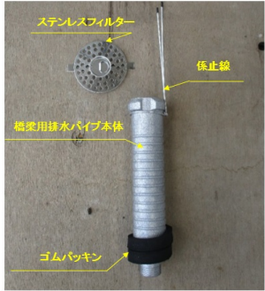
鉄心管（いしんかん）「橋梁用排水パイプ」の各部品名称
