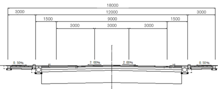
交差点部
