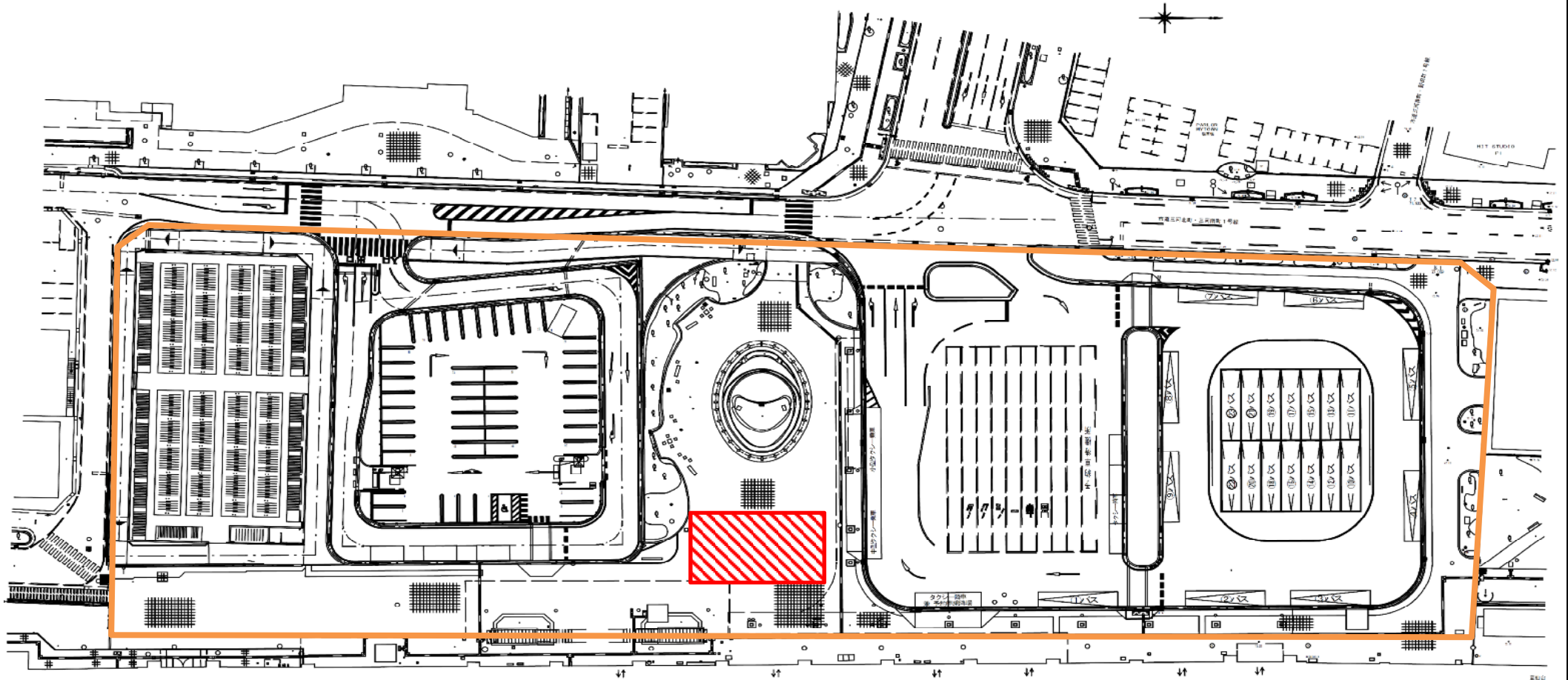
福島駅西口駅前広場レイアウト
