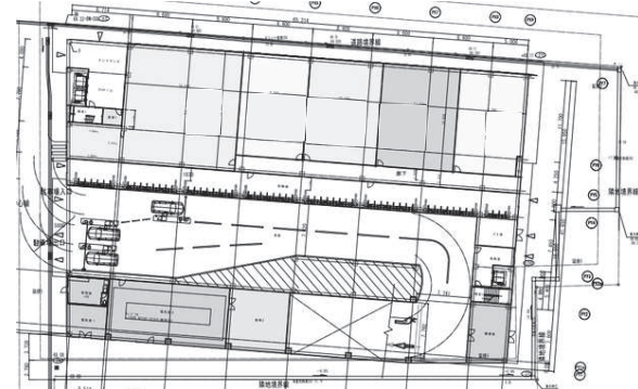
▲ 駐車場棟平面図
