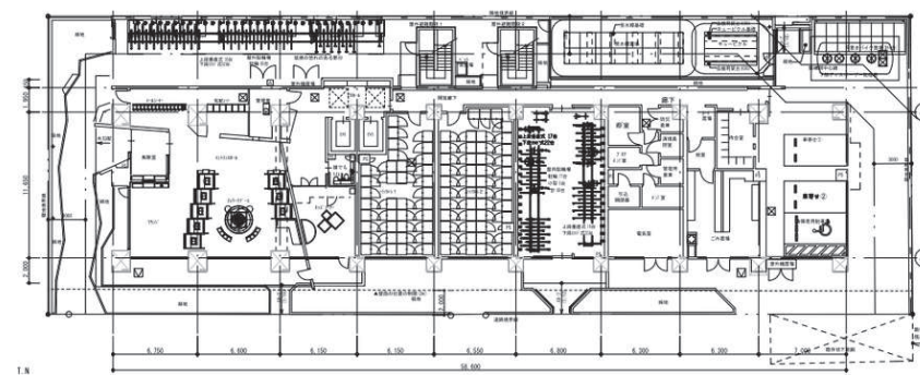
▲ 住宅棟平面図
