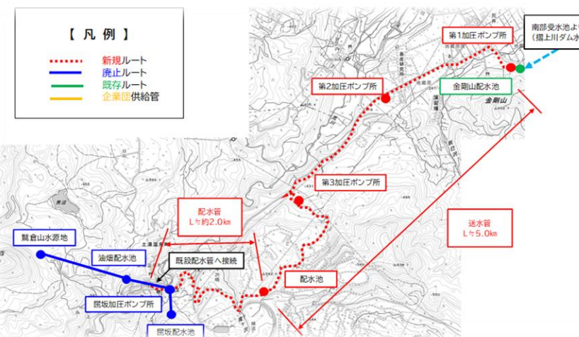
土湯地区水道施設整備事業の概要（イメージ）
