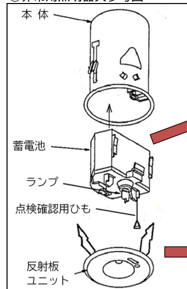
③非常用照明器具参考図
