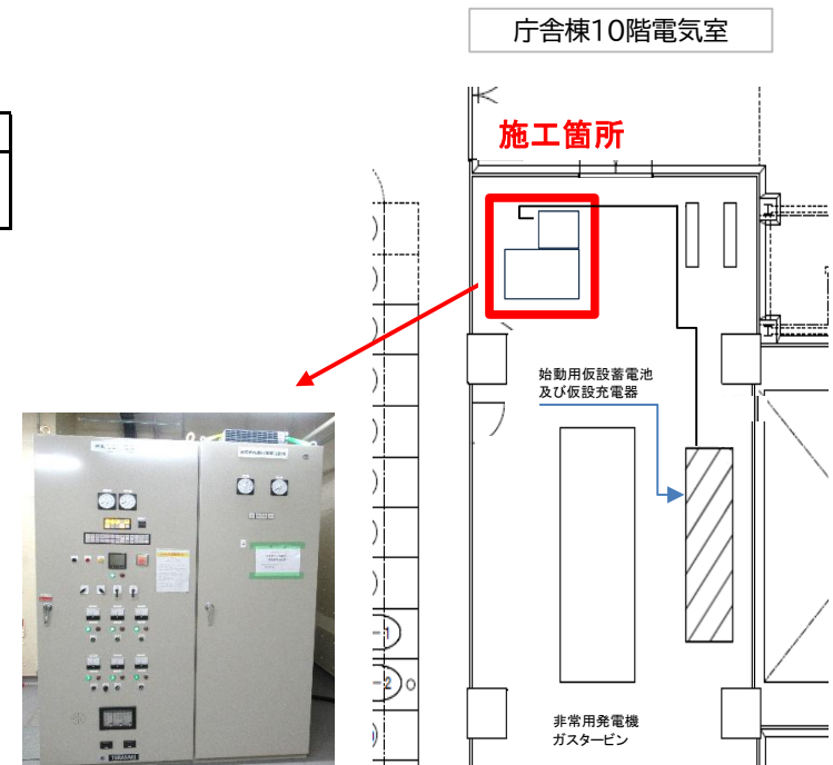
右：始動用直流電源装置
