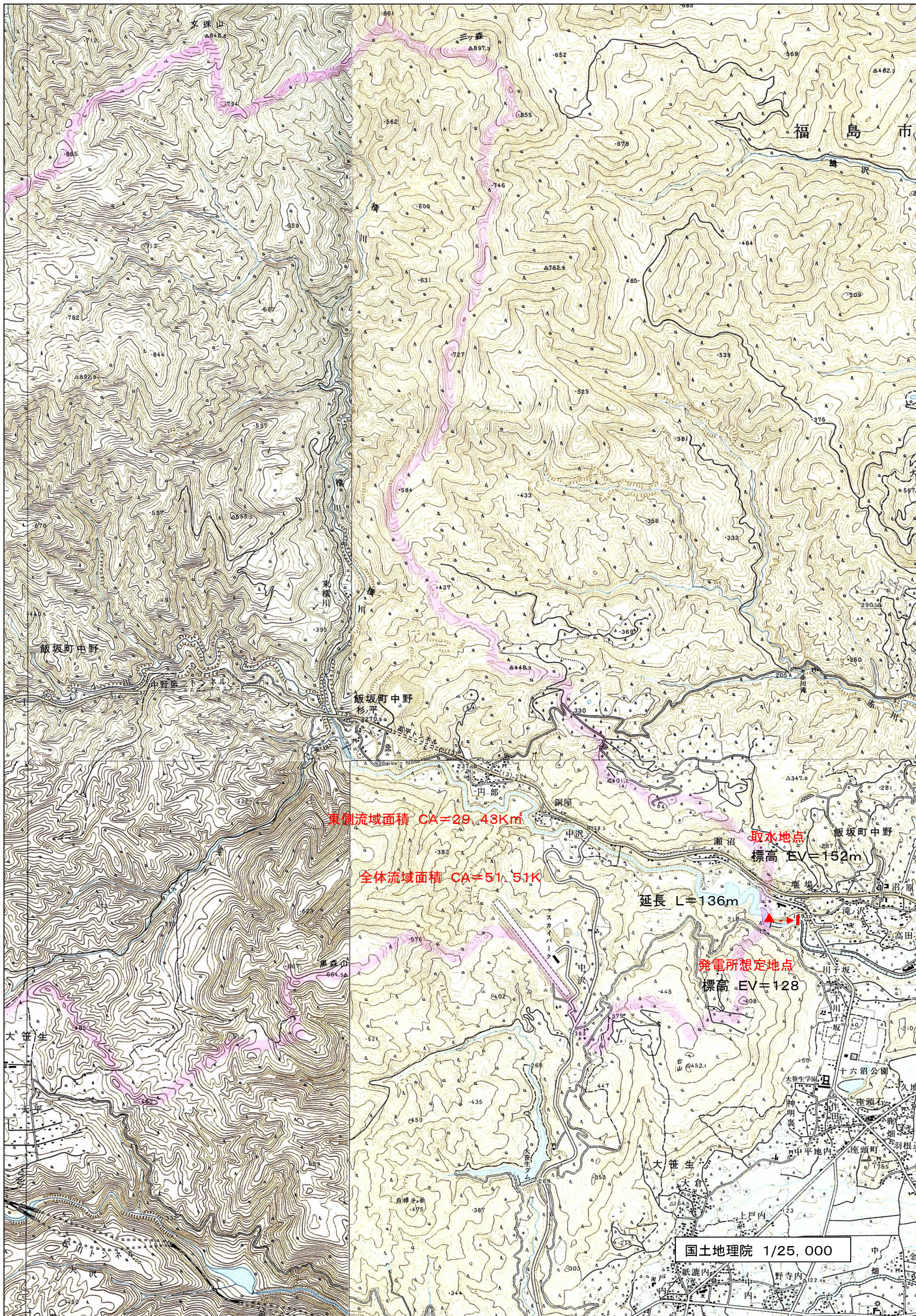
4-1 発電所想定位置及び流域面積図 ①
