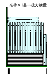
枠NSF-89×10基 床板NF-9D×15枚
