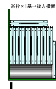
枠NSF-89×10基 床板NF-9D×15枚
