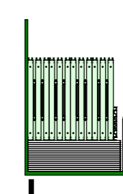
2枠一体型枠NSF-89W×4基 2段型ステップNSF-23S×1基 床板NF-9D×15枚
