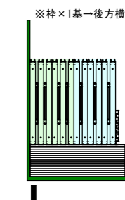
枠NSF-89×4基 2枠一体型枠NSF-89W×2基 2段型ステップNSF-23S×1基 床板NF-9D×15枚
