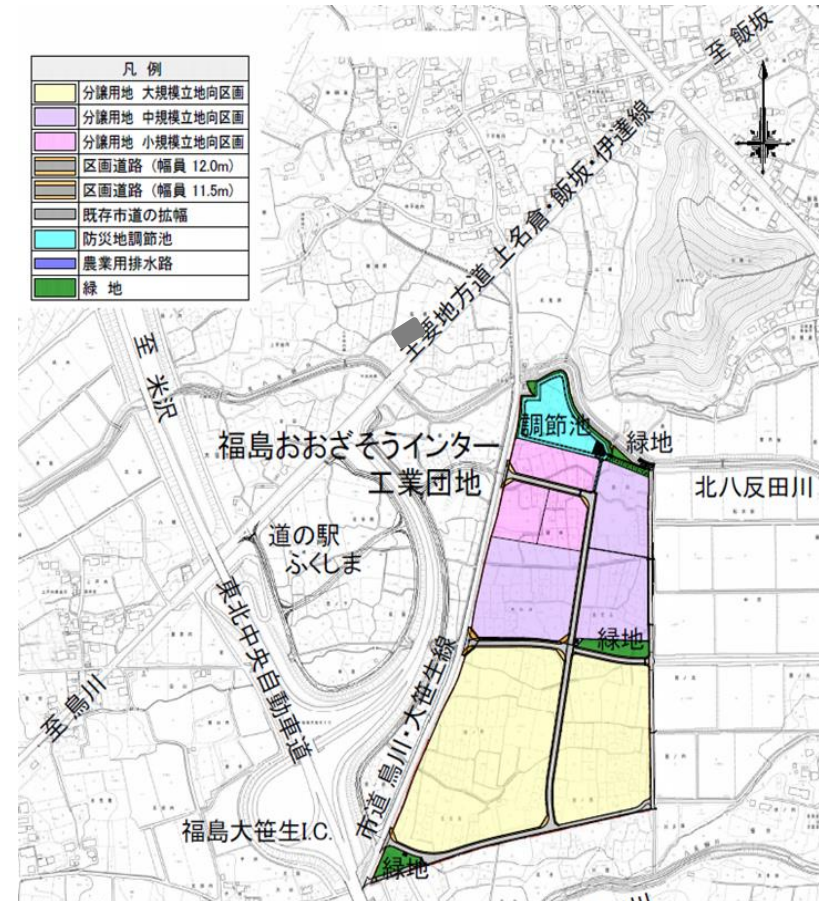
第2期分譲計画図(分譲8区画)
