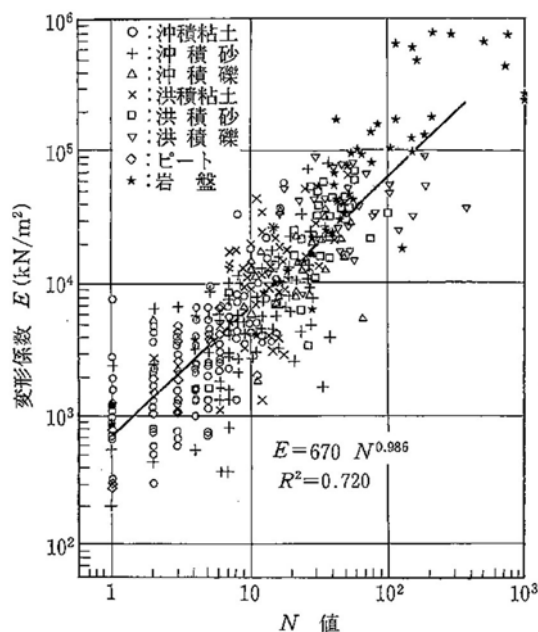
図 4.2.3 孔内水平載荷試験より得られた変形係数と N 値との関係 (土砂)
