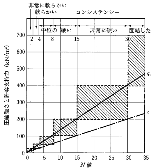
図 4.2.1 N値と粘土のコンシステンシー、一軸圧縮強さ及び許容支持力との関係 (Terzaghi, Peck)
