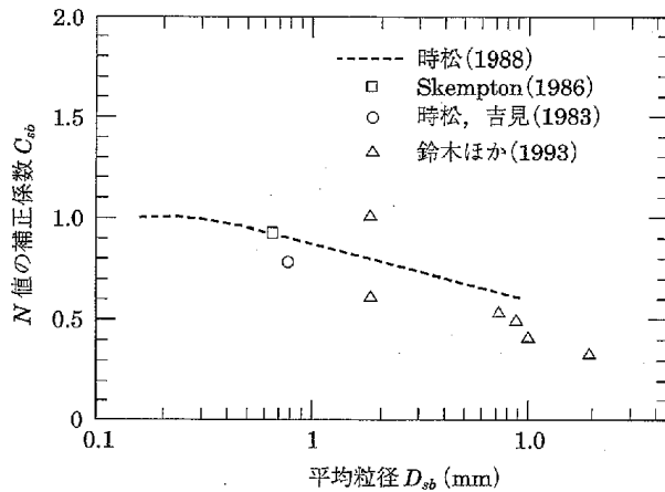
図 4.5.4 砂礫地盤の N 値補正係数 4.5.3)
