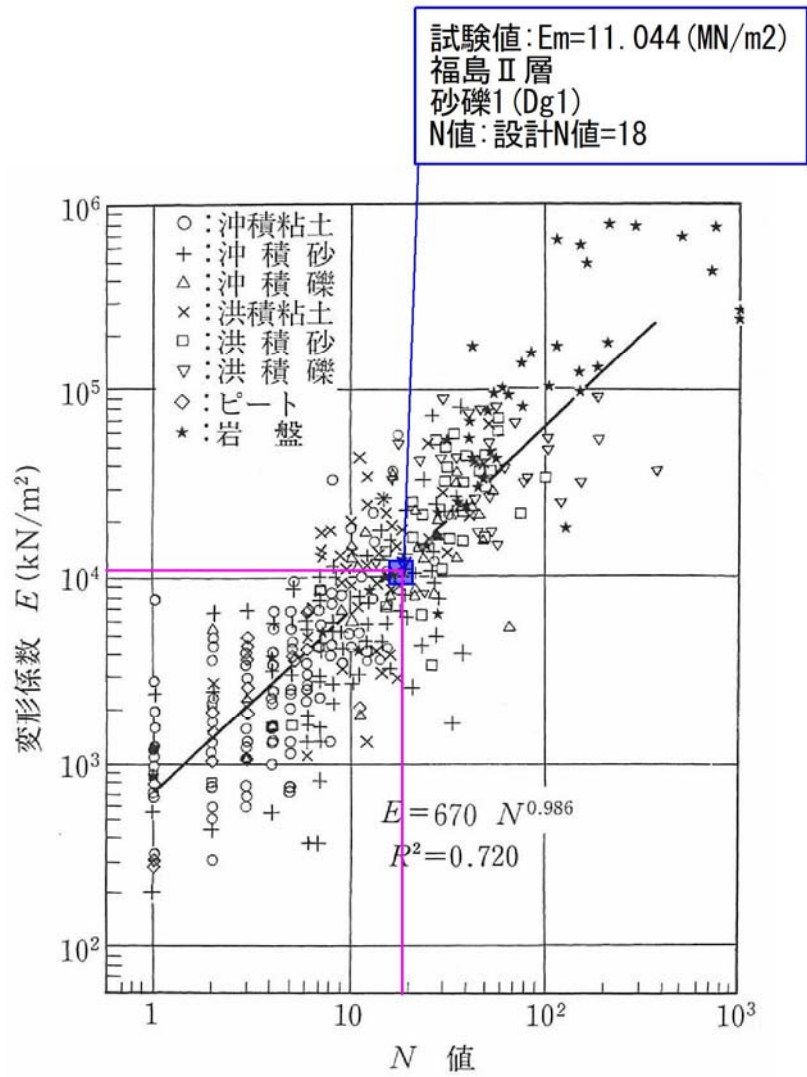
図 3.6.1 孔内水平載荷試験より得られた変形係数と N 値との関係 (地盤工学会：地盤調査の方法と解説，P687，平成 25 年 3 月)
