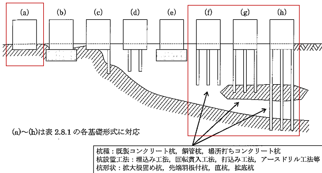
図 4.4.1 支持地盤の深度と適応可能な基礎形式
