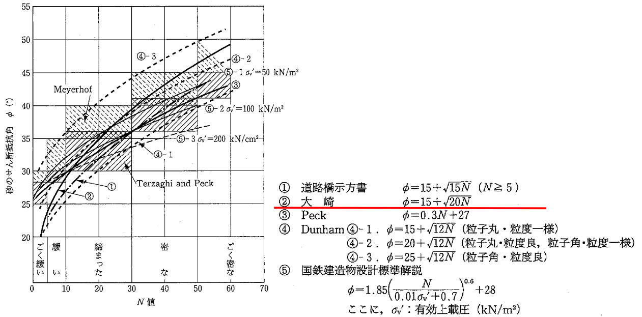
図 4.2.2 N 値と砂のせん断抵抗角の関係
